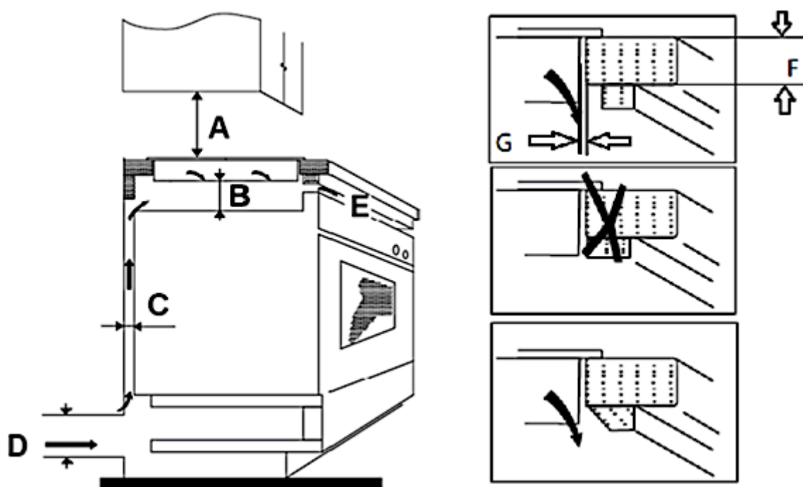
C = BELÜFTUNGSSCHLITZ
